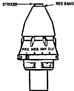
U AR4488-A Armed fuze.
