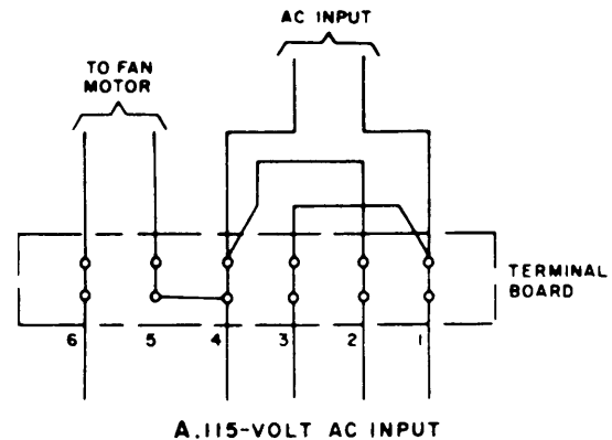
A. 115-VOLT AC INPUT
