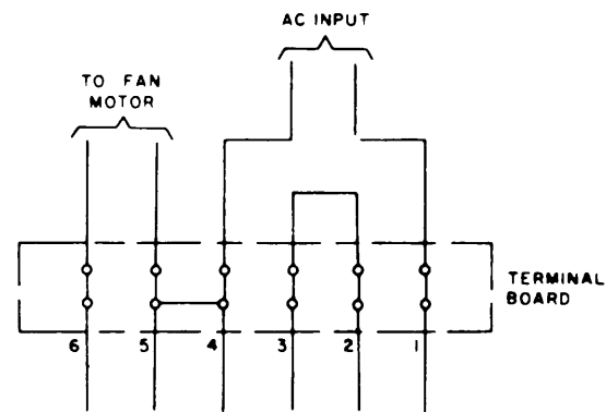
B. 230-VOLT AC INPUT
