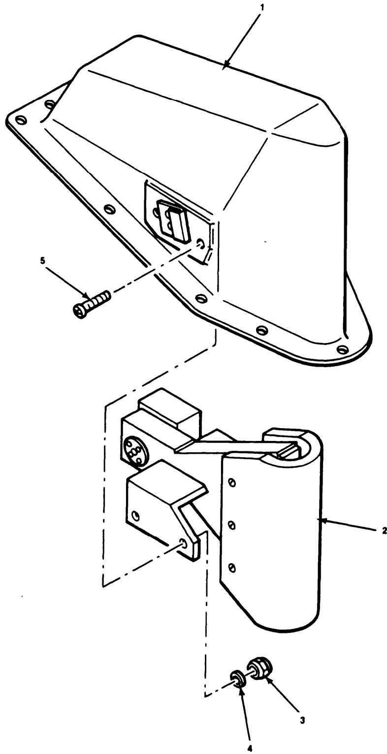
Figure 2. Antenna AS-3007/ALQ-136(V).
