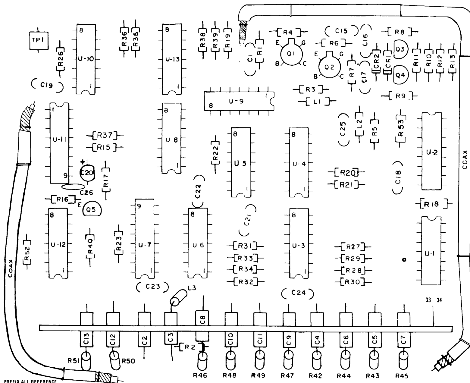
4-27 VHF Divider (CCA)
