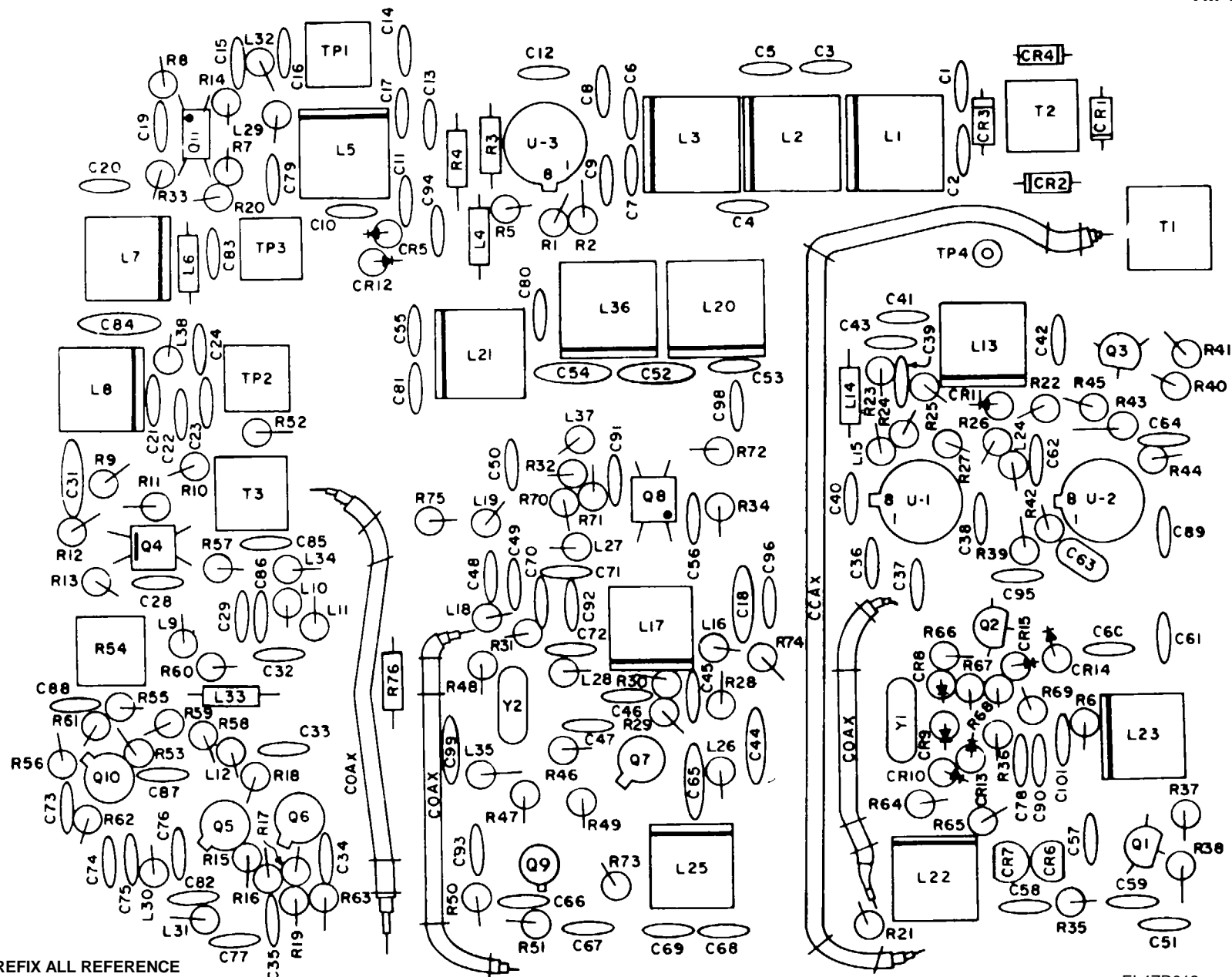
4-26 Translator(CCA)
